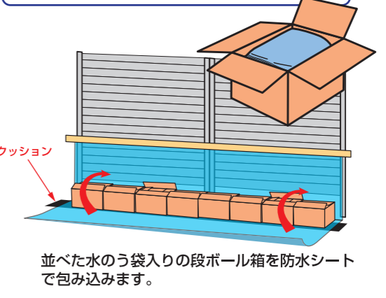
止水クッションをグラウンド面に敷いてから防水シートの上に水のう袋を積み上げます。グラウンド面と防水シートの隙間を出来るだけ少なくします。 積み上げた水のう袋を防水シートで包み、耐水テープなどで防水シートを固定します。
