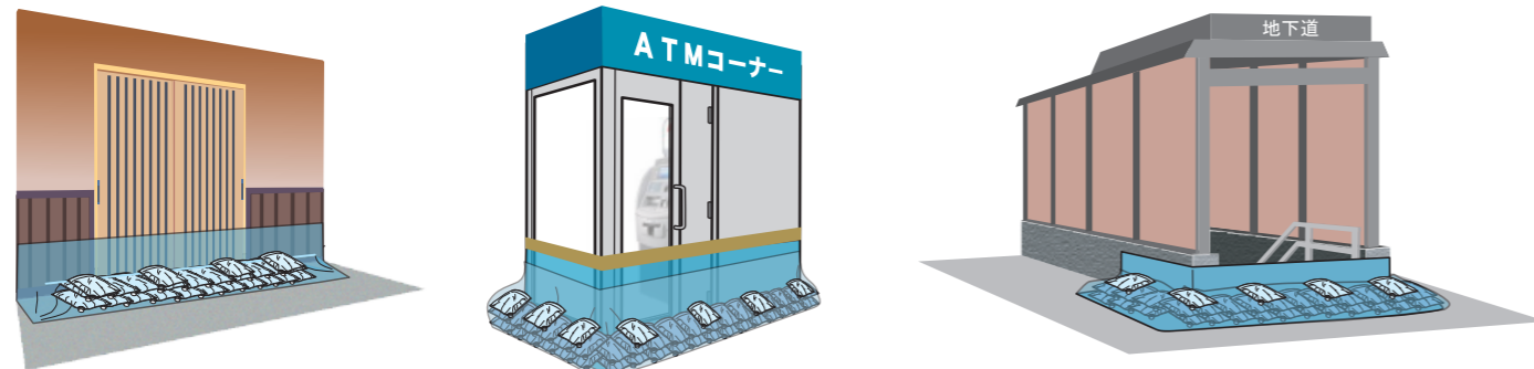
1.8m (1 間) 幅の玄関など 3 段積みの場合 水のう袋 約 30 袋 防水シート 幅約 4m～ 止水クッション 2m 屋外 ATM ブースなど 2 段積みの場合 水のう袋 約 30～50 袋 防水シートに包んでください。 地下道出入口など 2 段積みの場合 水のう袋 約 30～40 袋 防水シート 幅約 5m～10m
